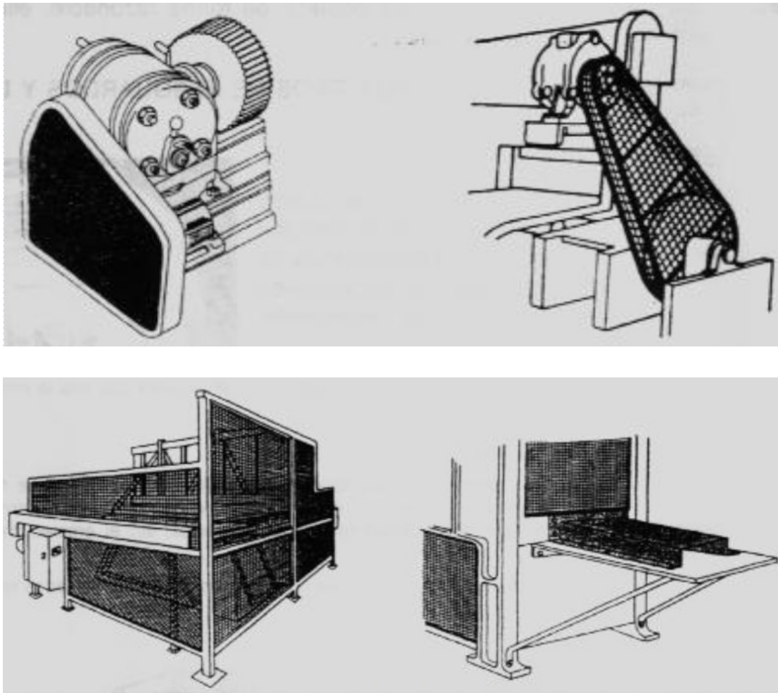
Algunos ejemplos de resguardos fijos. Fuente: Norma UNE EN 953
