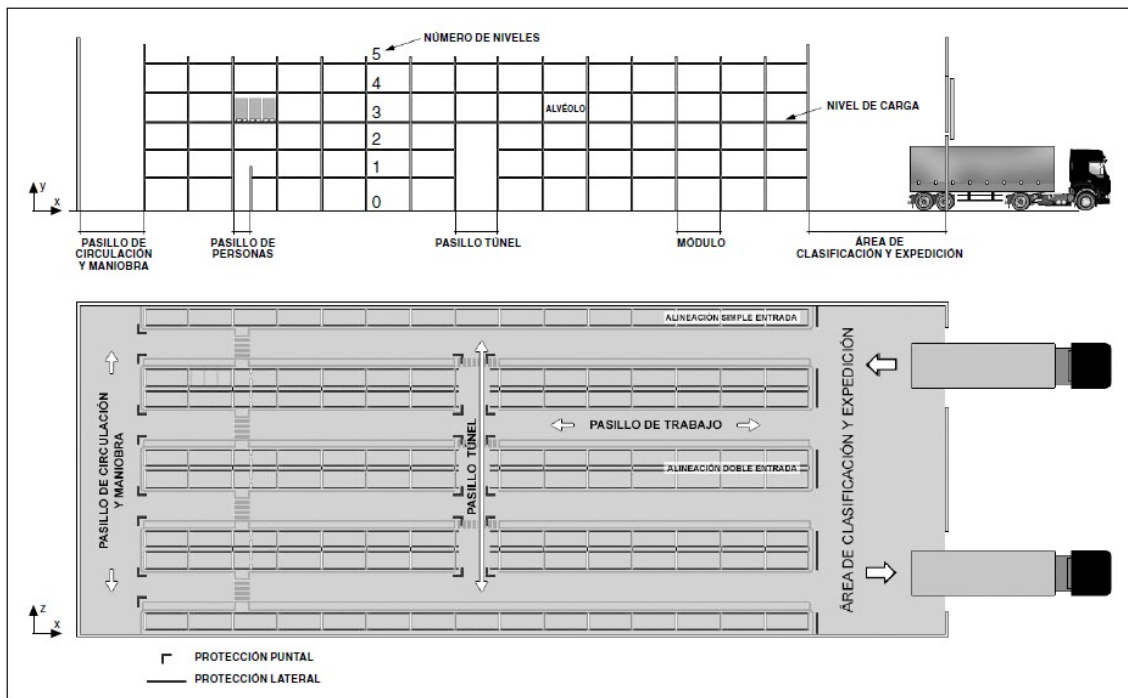
Ordenación adecuada de almacén. Fuente: NTP 852. Instituto Nacional de Seguridad e Higiene en el Trabajo
