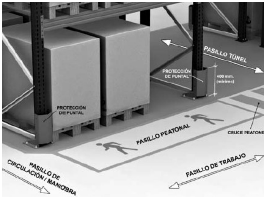
Protección de estanterías. Fuente: NTP 852. Instituto Nacional de Seguridad e Higiene en el Trabajo
